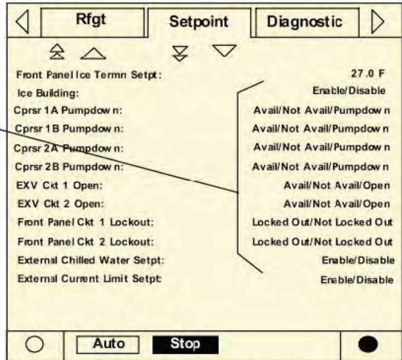
Tela de Set point - Parte Intermediária
