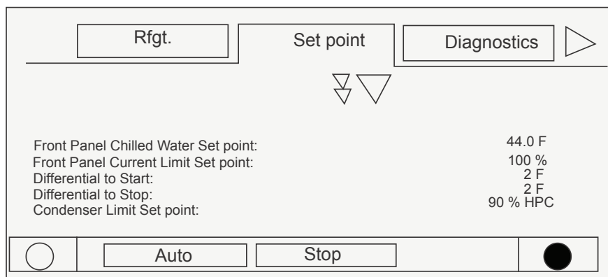
Tela de Set point - Parte Superior
