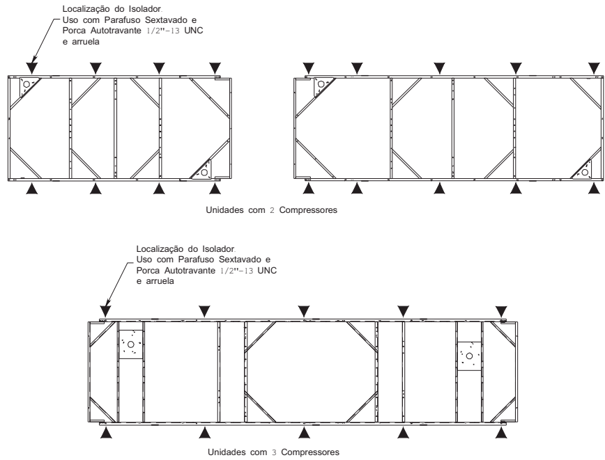
Fig. III-04 - Isolamento da Unidade
