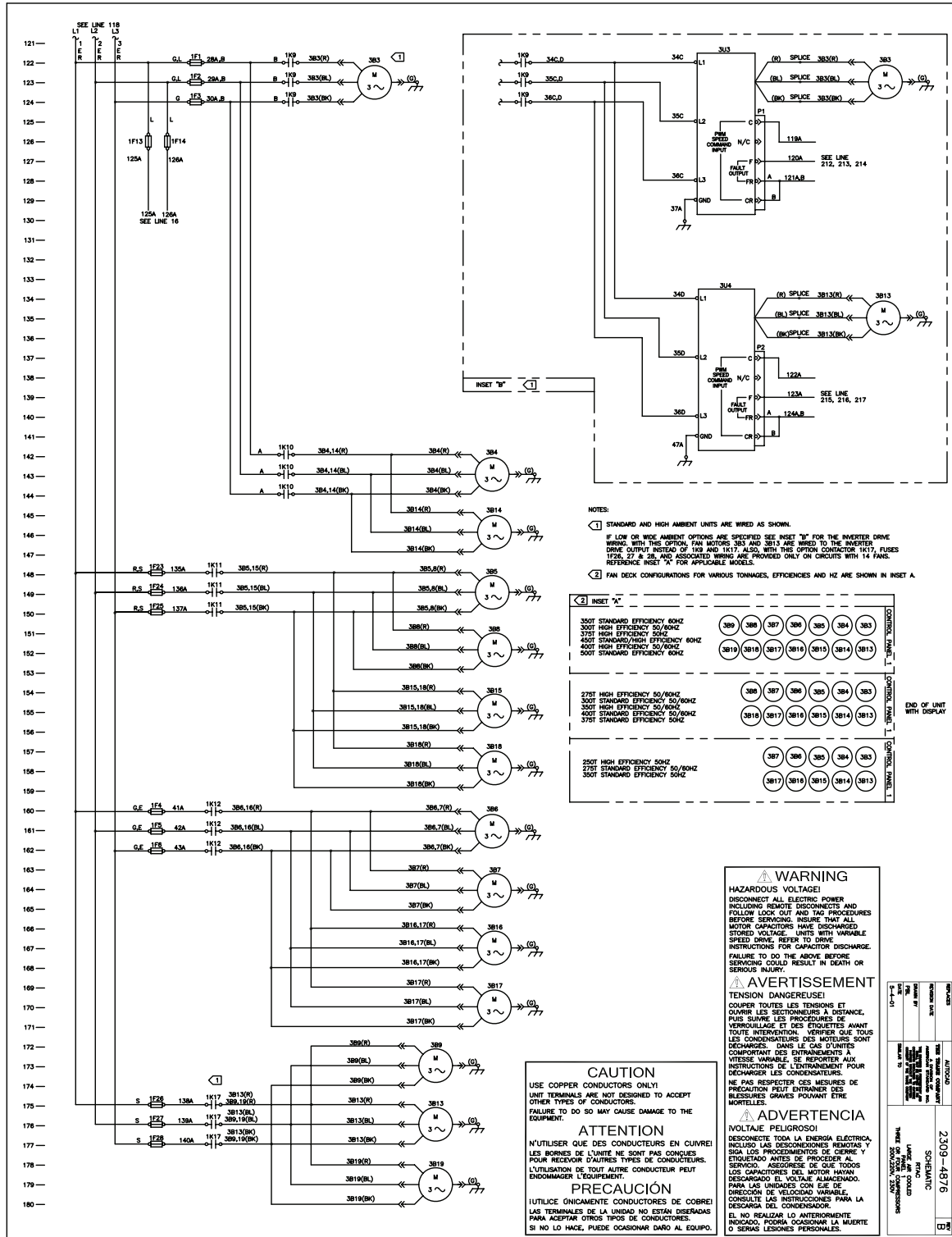
Fig XII-10 - Esquema Eléctrico, Vent, 3&4 Comp, Circuito1, Baixa Tensão
