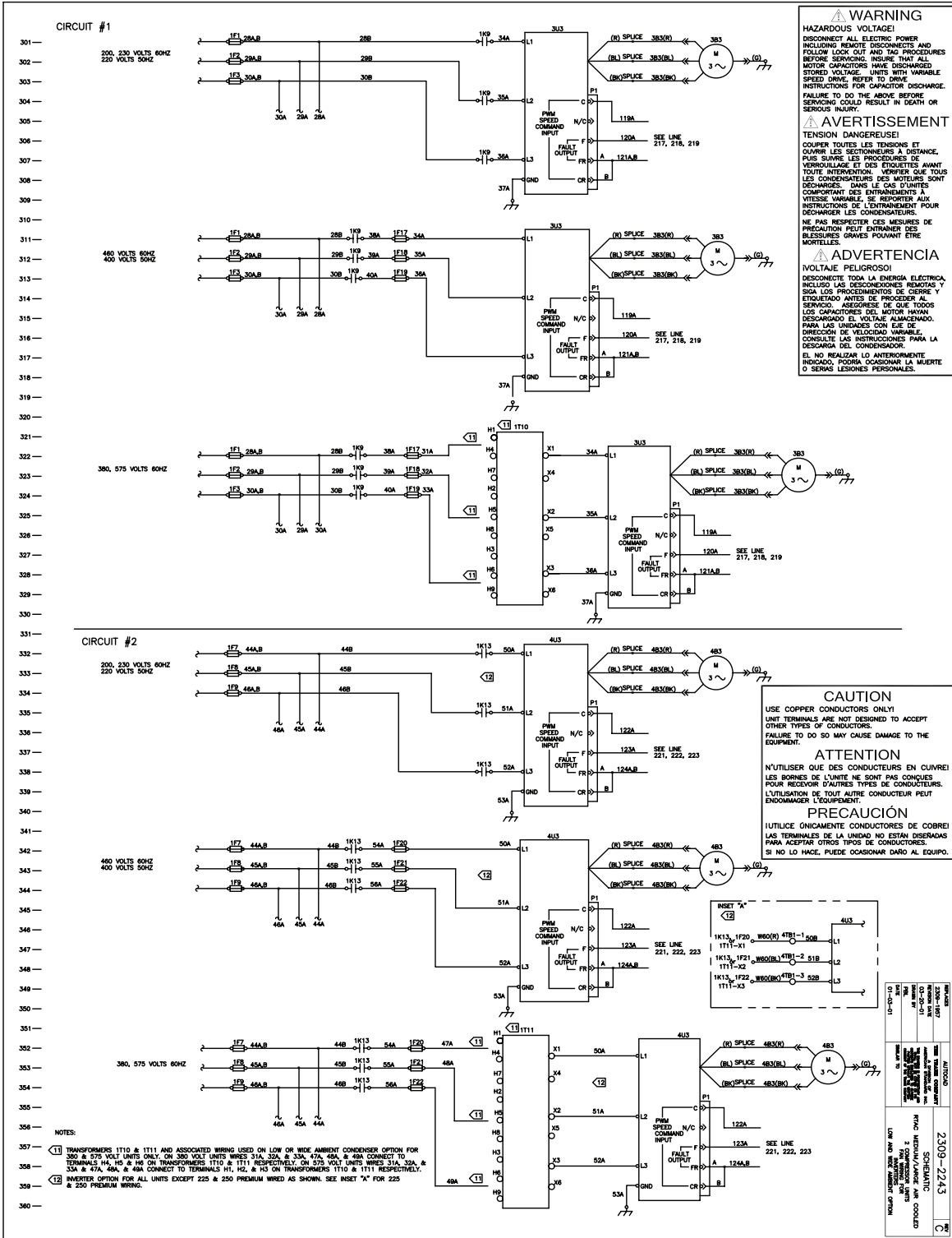
Fig XII-18 - Esquema Eléctrico, Vent, M&L, Inverters
