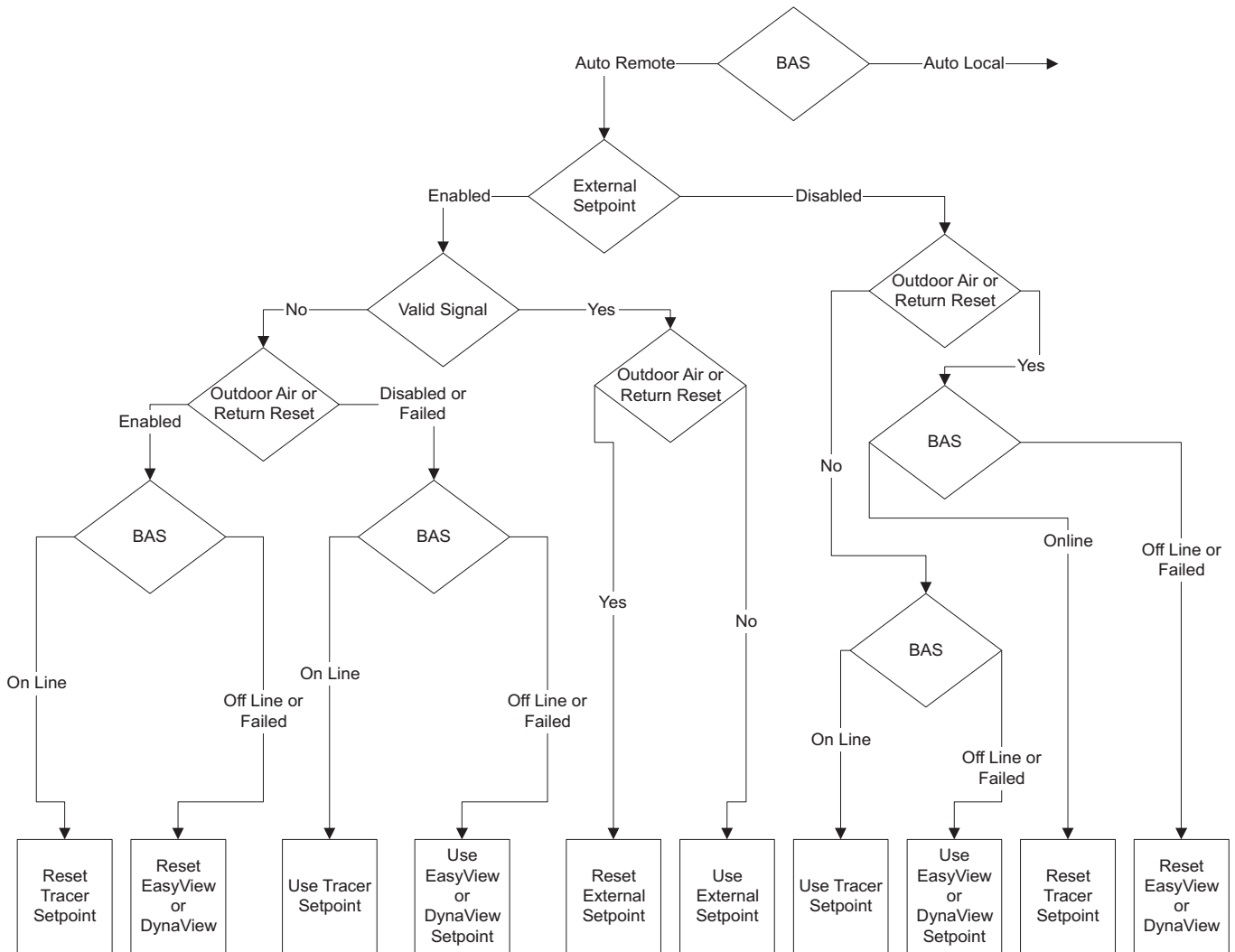
Fig. IV-05 - Fluxogramas de Arbitragem de Pontos de Configuração da Água Refrigerada (Auto Remoto)
