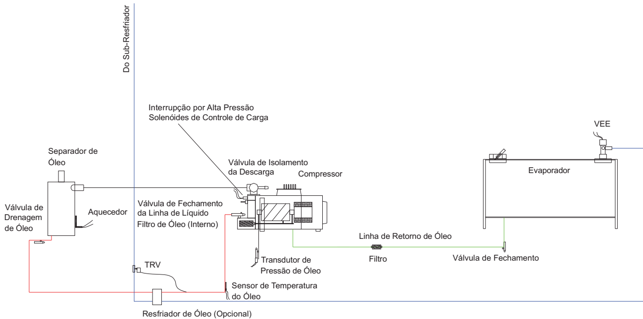
Fig. XI-01 - Diagrama Esquemático do Sistema de Óleo
