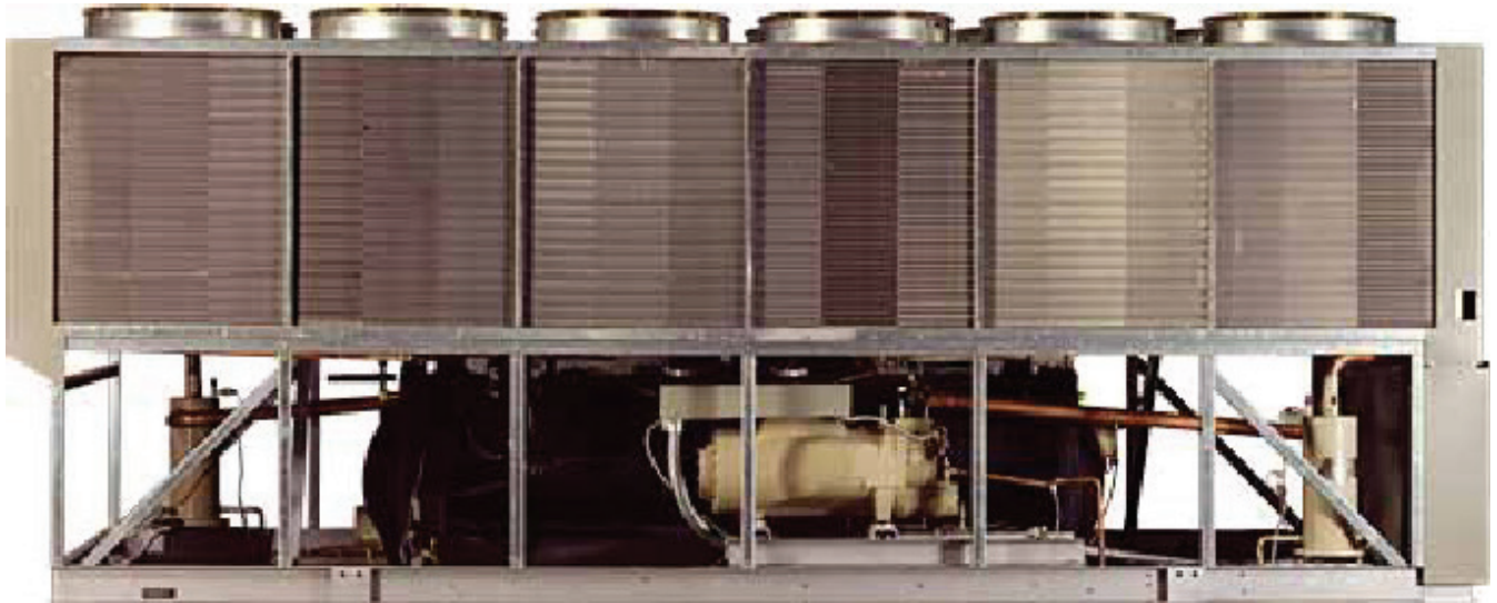
Fig. II-02 - As fotografias a seguir mostram o RTAC em duas vistas.
