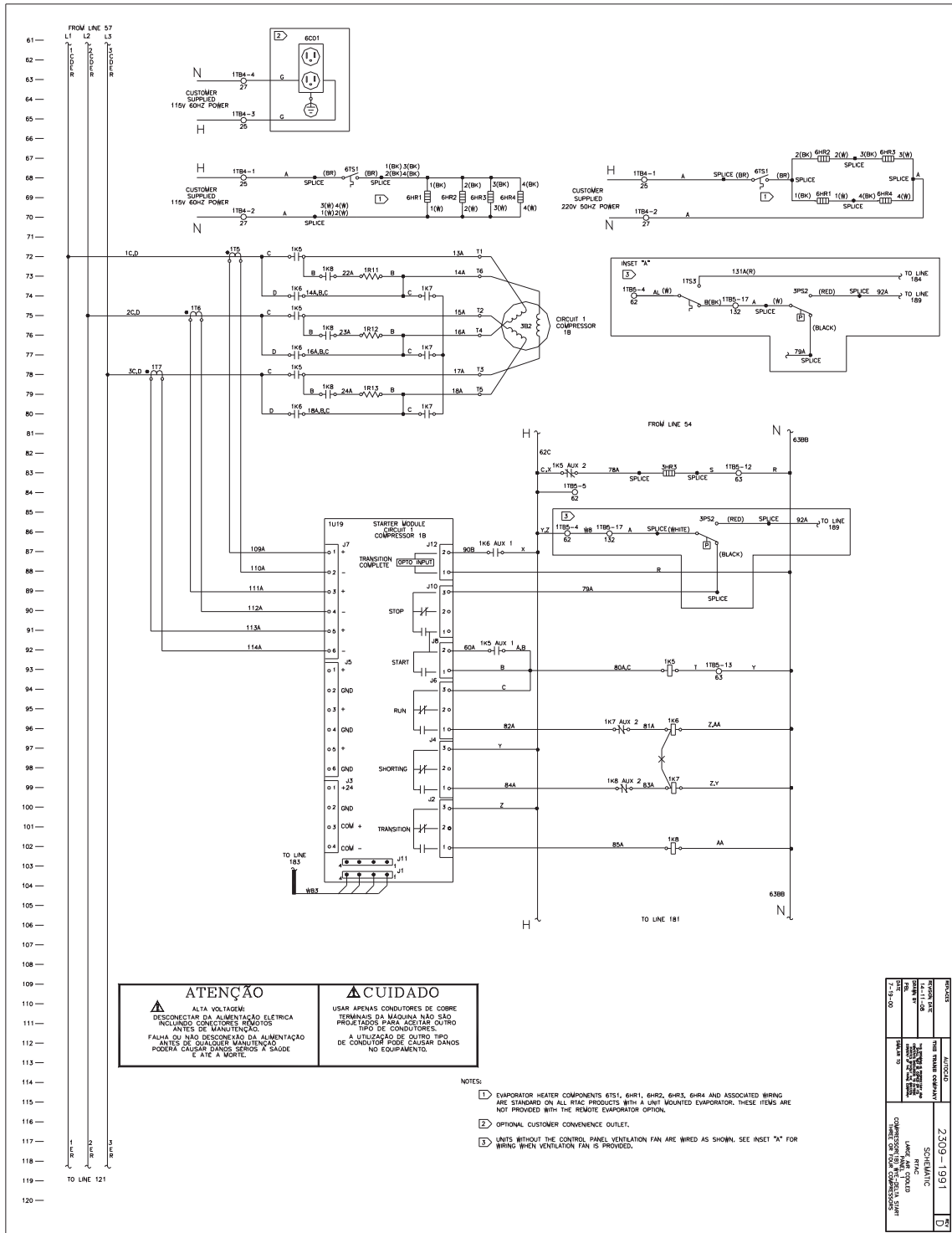
Fig XII-04- Esquema Elétrico, 3&4 Comp, Comp 1B, Y-D
