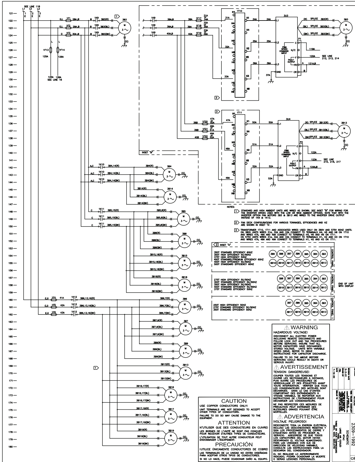
Fig XII- 11 - Esquema Elétrico, Vent, 3&4 Comp, Circuito1, Alta Tensão
