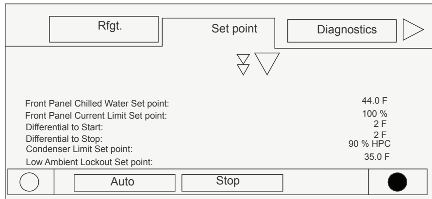
Tela de Stepoint - Parte Superior
