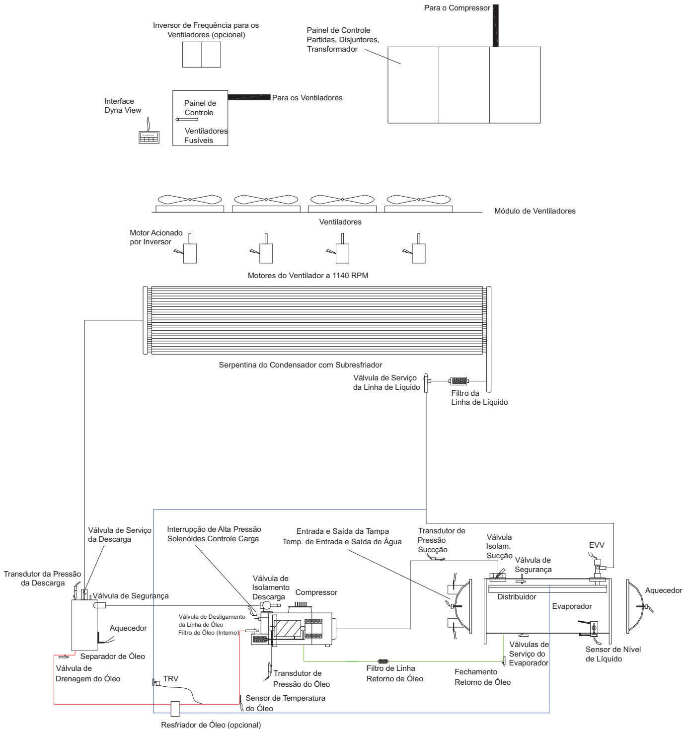
Fig. V-02 - Desenho esquemático do sistema
