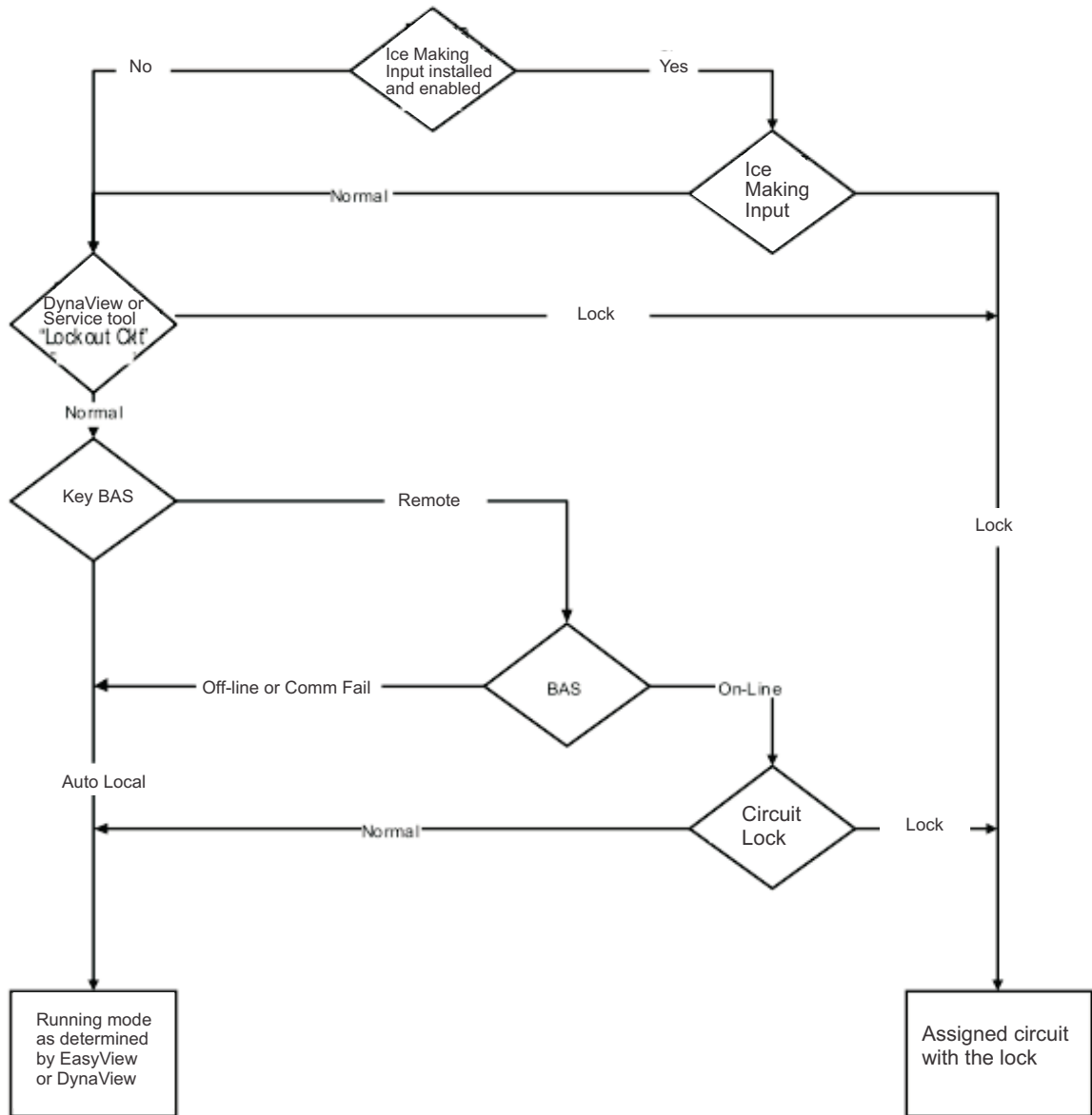
Fig. IV-08 - Fluxogramas de Arbitragem de Pontos de Configuração de Bloqueio do Circuito
