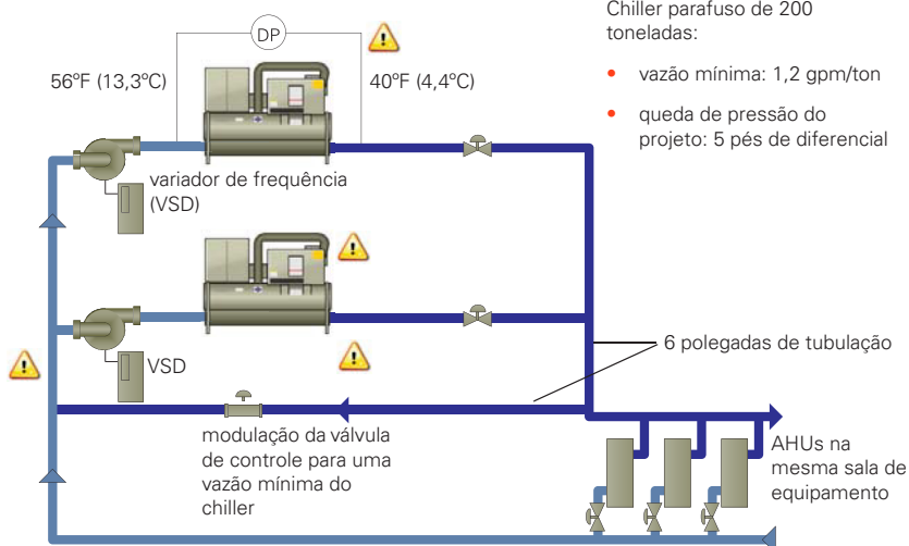
Figura 1. Caso 1: Nova vazão primário variável (VPF)
