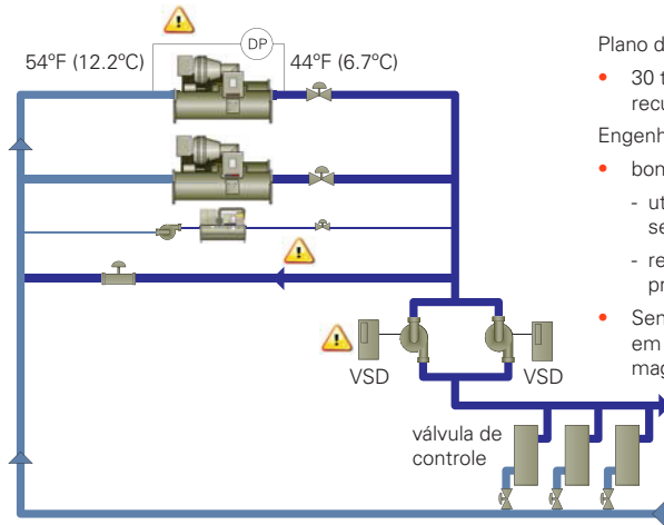
Figura 3. Caso 2: Após a conversão de valor em VPF
