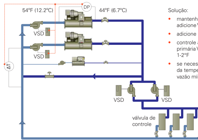
Figura 4. Conversão para variável primária-variável secundária
