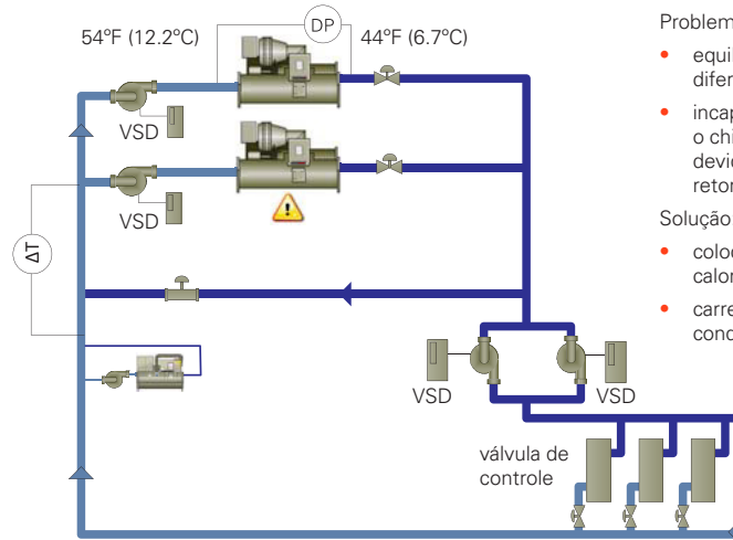
Figura 1. Caso 1: Nova vazão primário variável (VPF)
