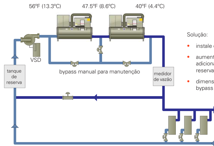
Figura 2. Novos chillers da série da vazão primária variável (VPF)
