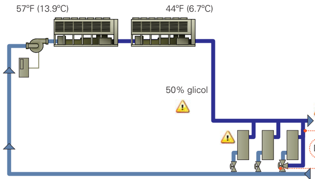
Figura 6. Modernização de chillers da série VPF
